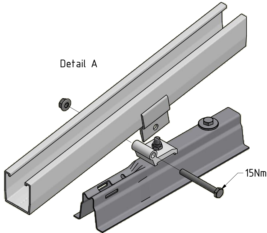
Subassembly profile
